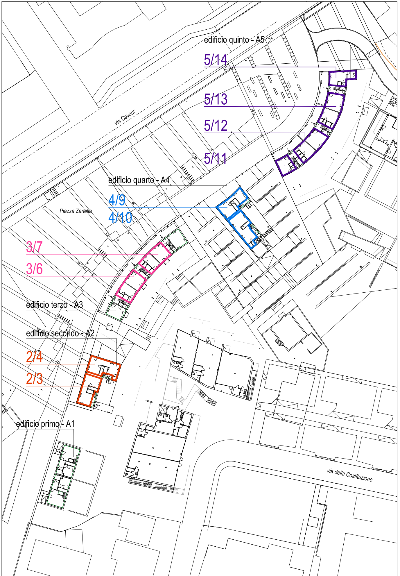
Planimetria dei piani terra del borgo rurale inseriti nel progetto approvato del 'Contratto di Quartiere'
