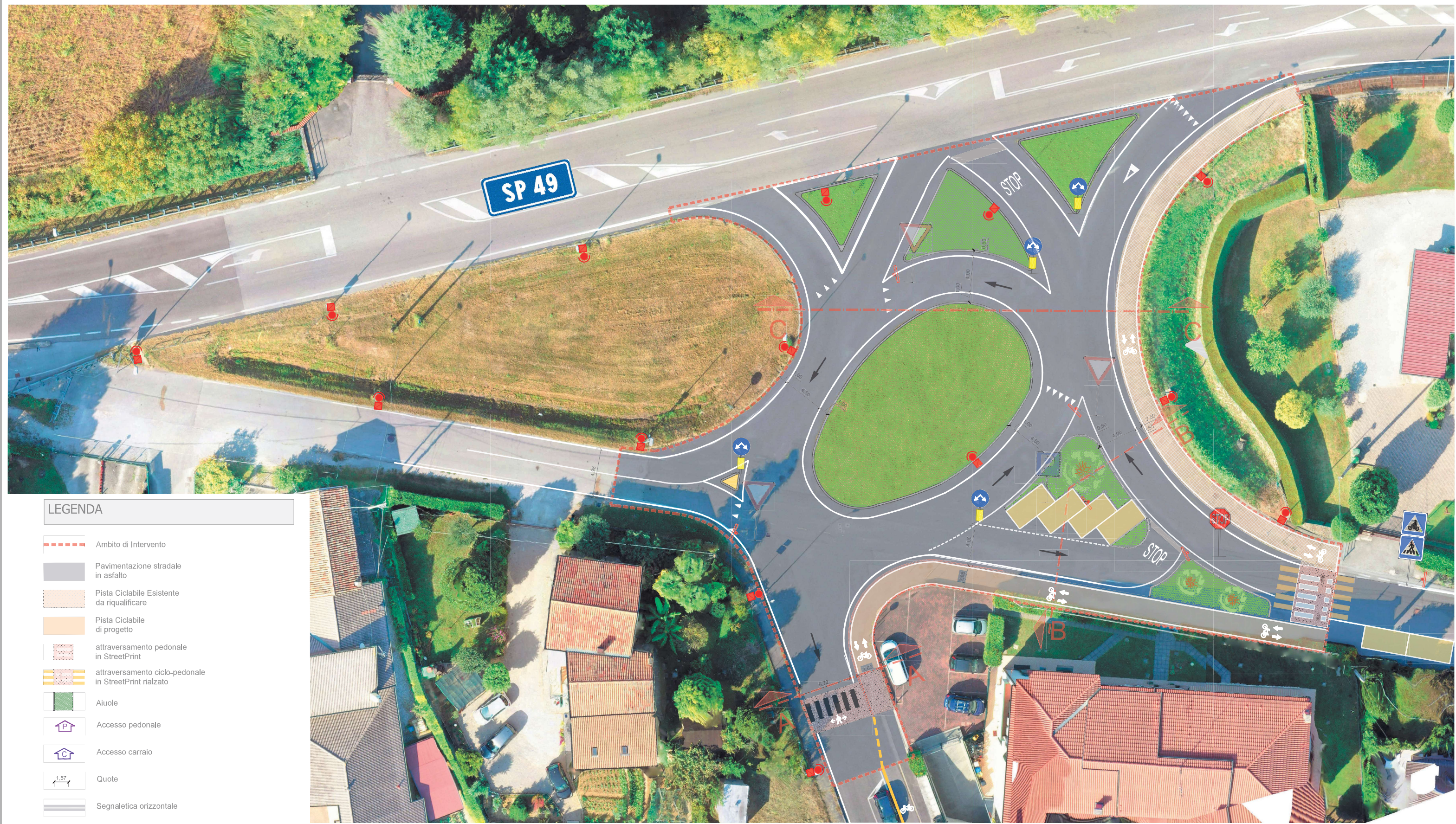
STATO DI PROGETTO - PLANIMETRIA GENERALE INCROCIO S.P. 49 - SUD scala 1:250
